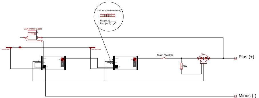
Abbildung 13. In Reihe geschaltete Batterien mit CAN-Netzkabel und externer Abschaltvorrichtung
