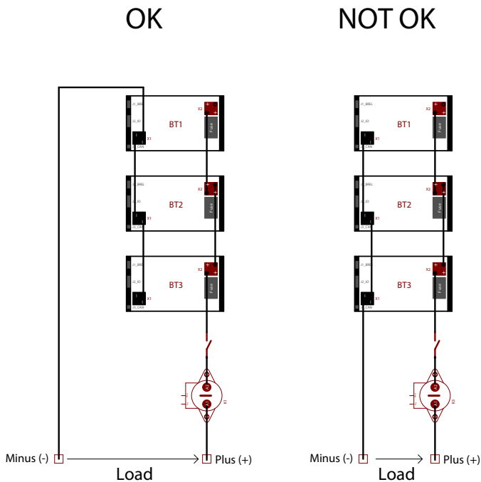
Abbildung 14. Drei Li-Ionen-Batterien parallel zur externen Abschaltvorrichtung
